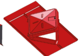
KATTOLUUKKU 600x600 mm
