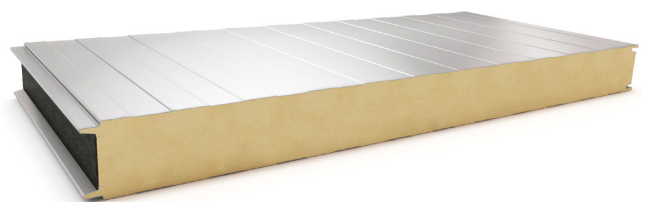
Seinäelementti PIR-120 mm U-arvo 0,19 W / m 2 K B-s1,d0, EI30
