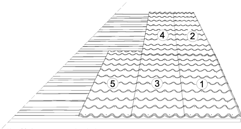
Kuva 20. Asennusjärjestys ja kiinniketiheys
