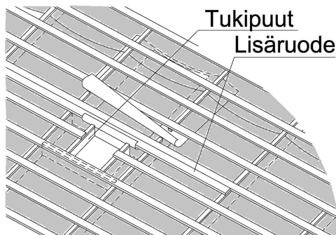
Kuva 13. Läpiviennin tuenta
