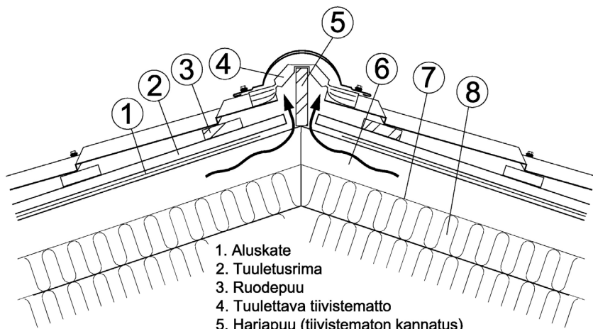
Kuva 12. Tuulettava harjan tiivistematto
