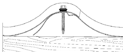
Kuva 17b. Oikein asennettu limitys
