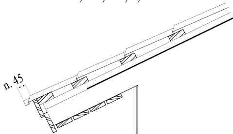
Kuva 15. Katelevyn räystääsyitys
