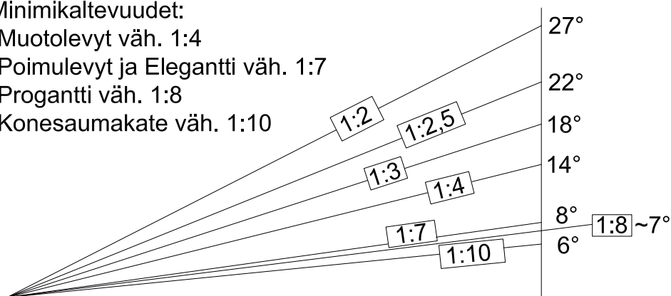
Kuva 27. Eri katetyyppien vähimmäiskaltevuudet
