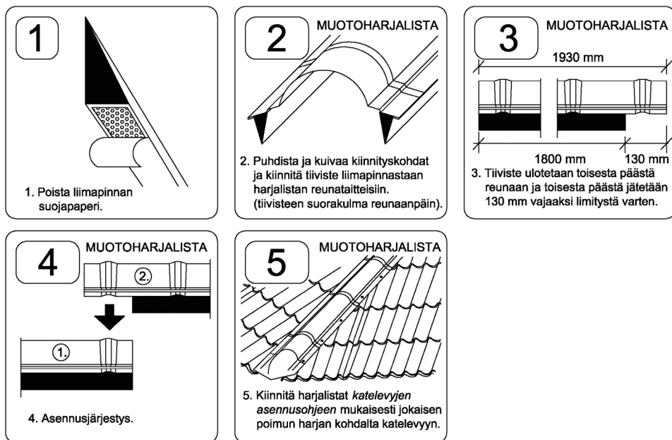
Kuva 28. Aumataitteen tiivistys
