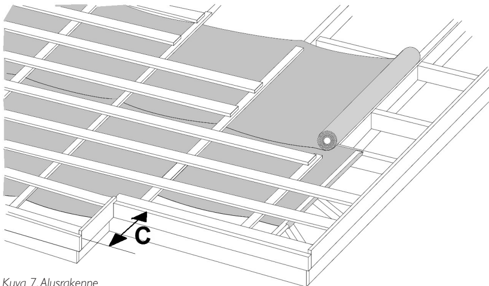
Kuva 7. Alusrakenne
