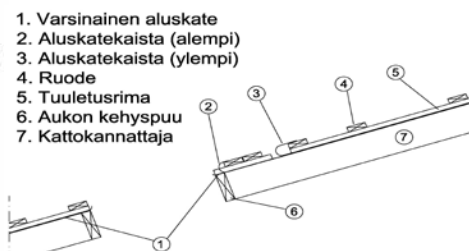
Kuva 9. Läpivientiaukkojen rakenteet
