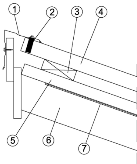
Kuva 19. Yläräystäs
