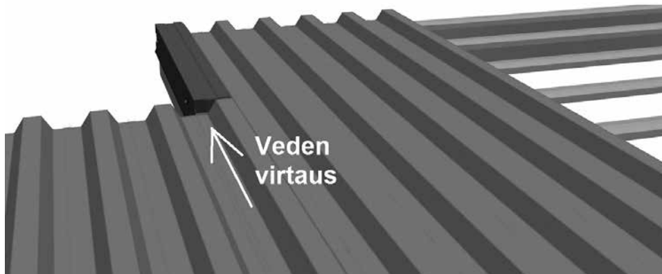
Kuva 14. Räystäälippa
