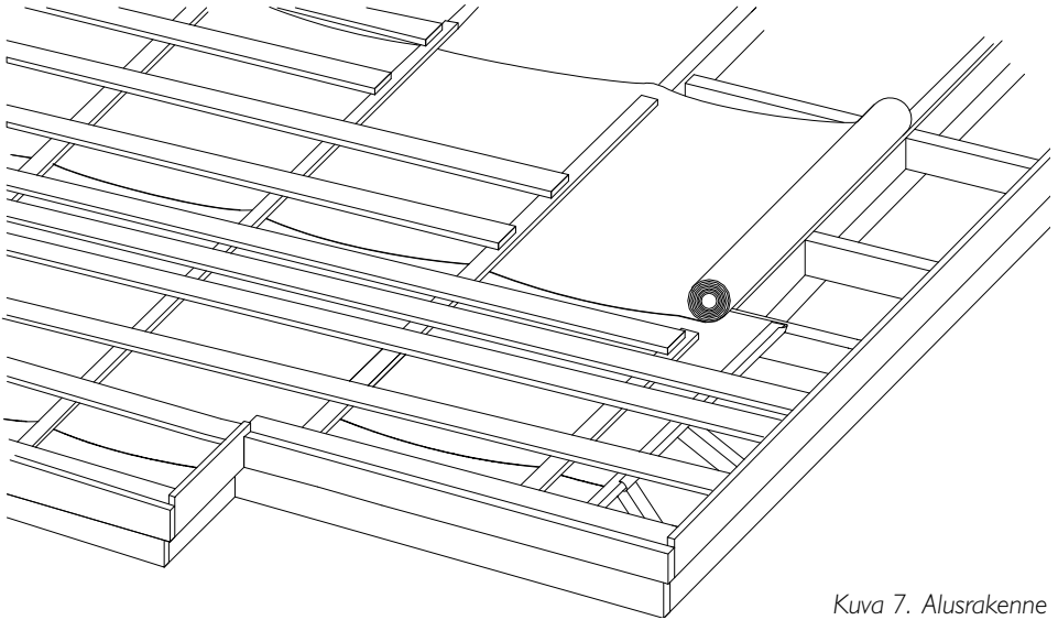
Kuva 7. Alusrakenne
