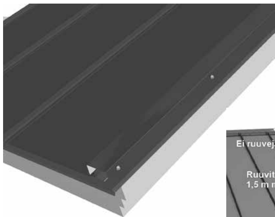
Kuva 24b. Päätilyistan kiinnitys ruoteeseen
