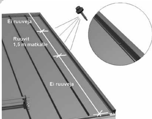
Kuva 24a. Päätilyistan kiinnitys päätilylataan
