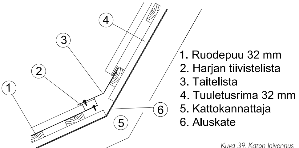
Kuva 39. Katon loivennus
