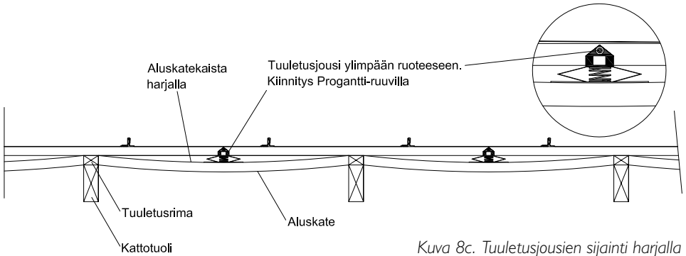
Kuva 8c. Tuuletusjousien sijainti harjalla
