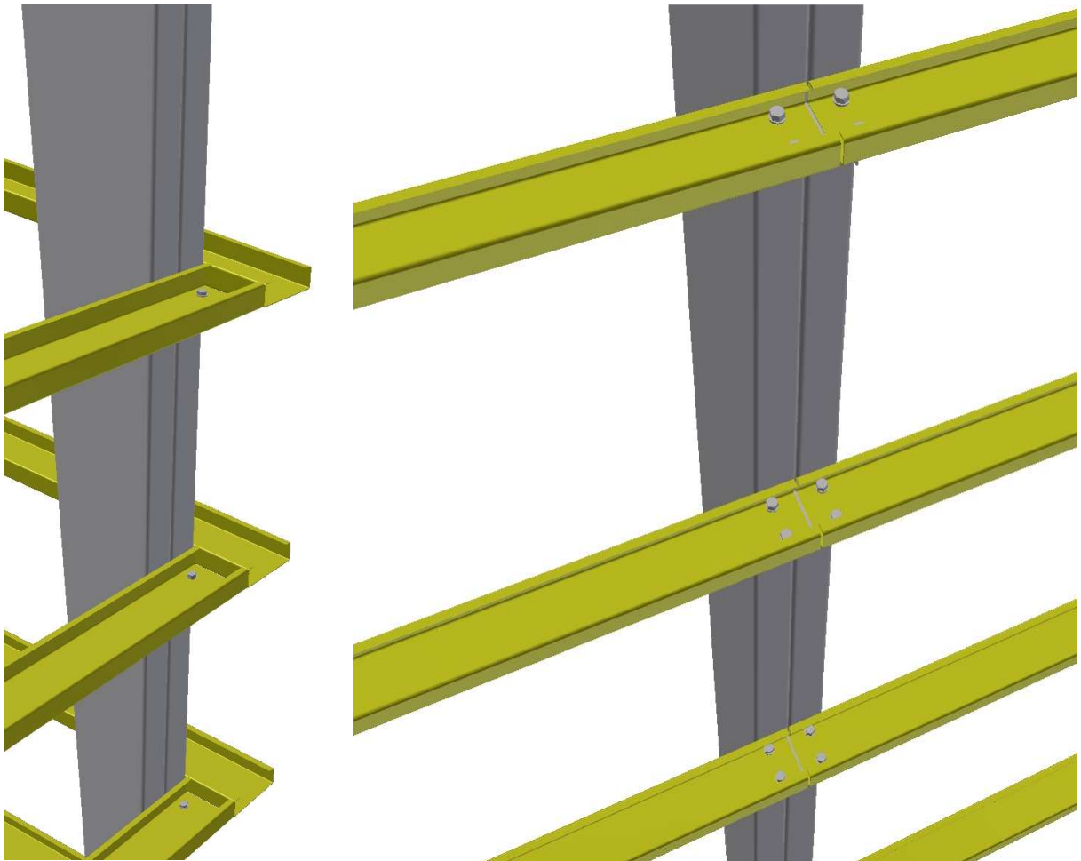
Kuva 23. C-orret seinässä, nurkka ja epäjatkuvuusliitos.
