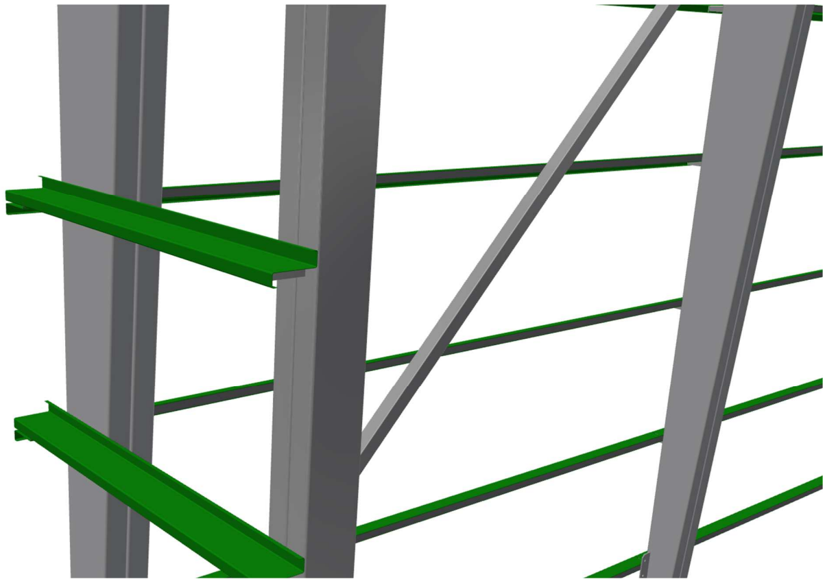
Kuva 22. Z-orret seinässä.
