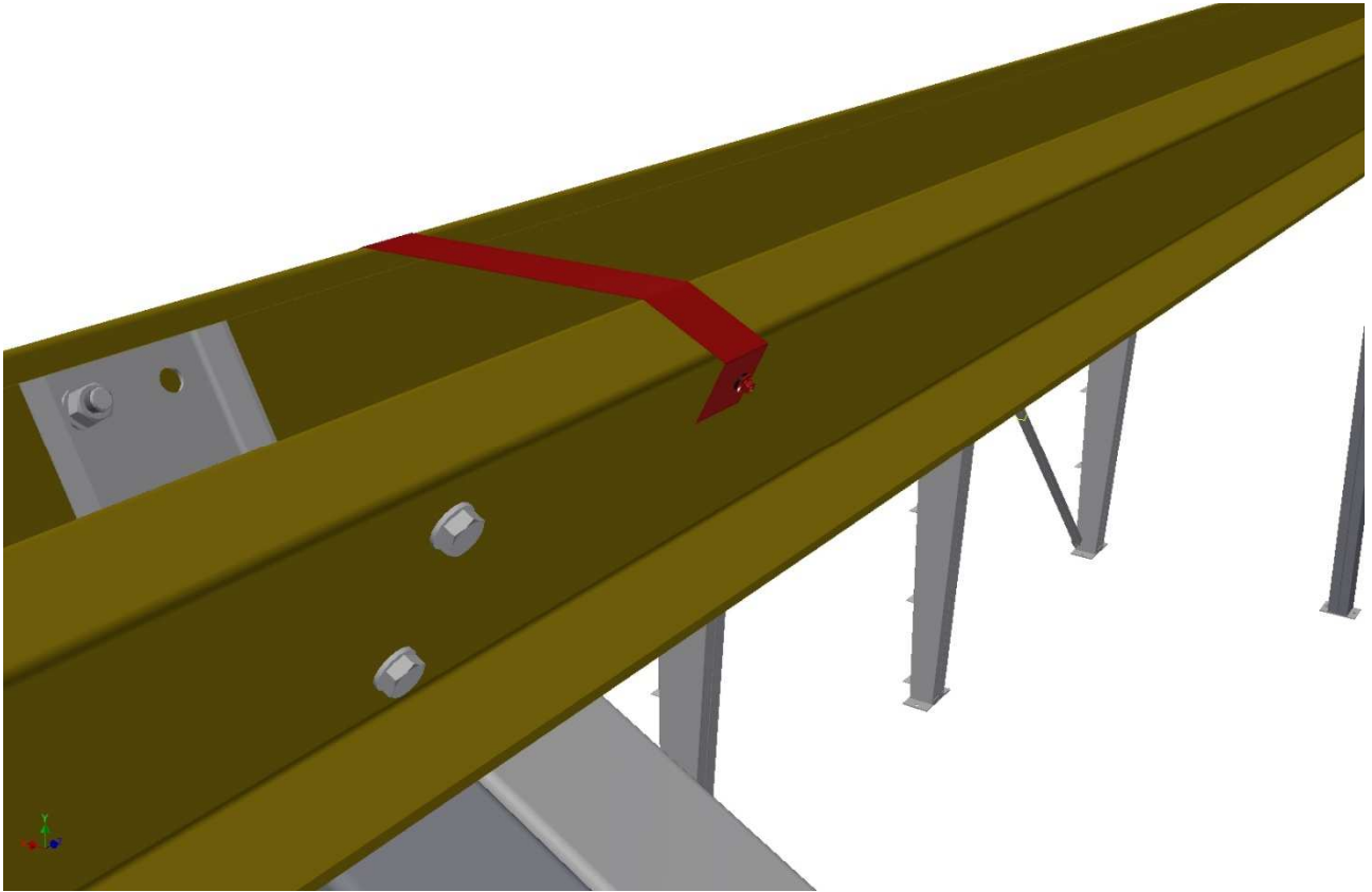
Kuva 21. Harjasidonta.
