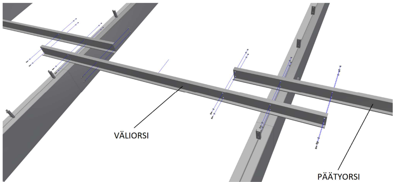
Kuva 18. Väliorren kiinnitys.
