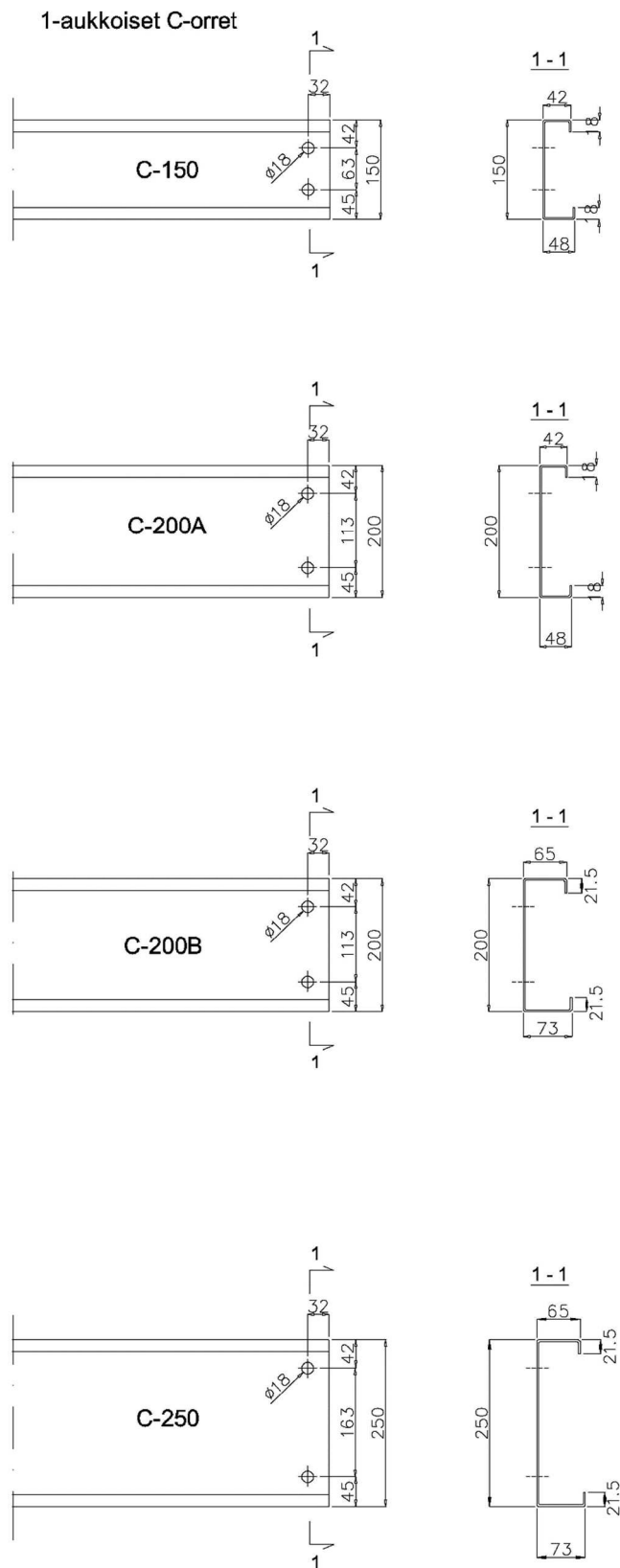
Kuva 2. C-orsien vakioreijitykset
