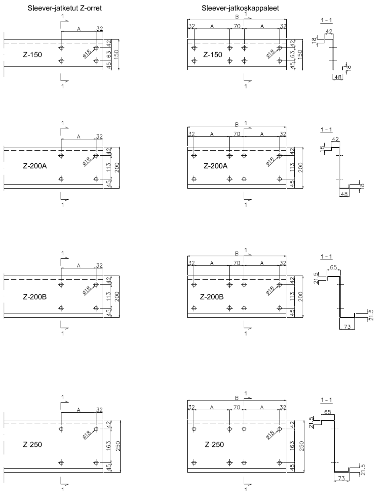
Kuva 4. Sivee-jatketujen Z-orsien vakioreijitykset.
