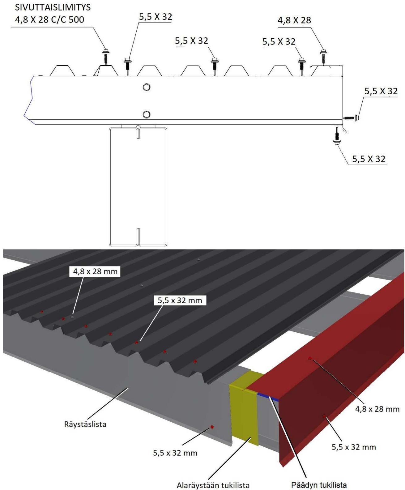
Kuva 24. Kattopellityksen kiinnitys kevytorsiiin.
