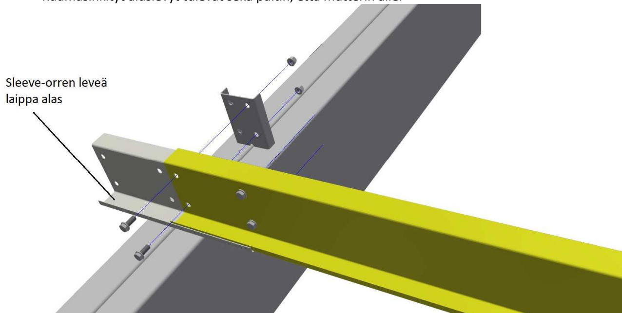
Kuva 19. Ensimmäisen katto-orren + Sleeve-orren kiinnitys.
