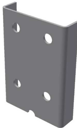
Kuva 7. Orsikiinnike teräspalkille.
