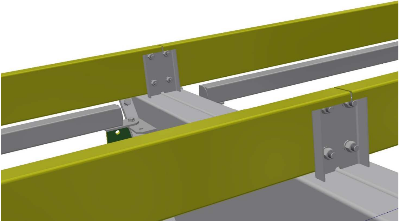
Kuva 11. Epäjatkuva orsiliitos.
