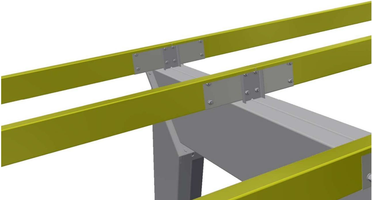
Kuva 13. Sleeve-jatkettu orsiliitos.
