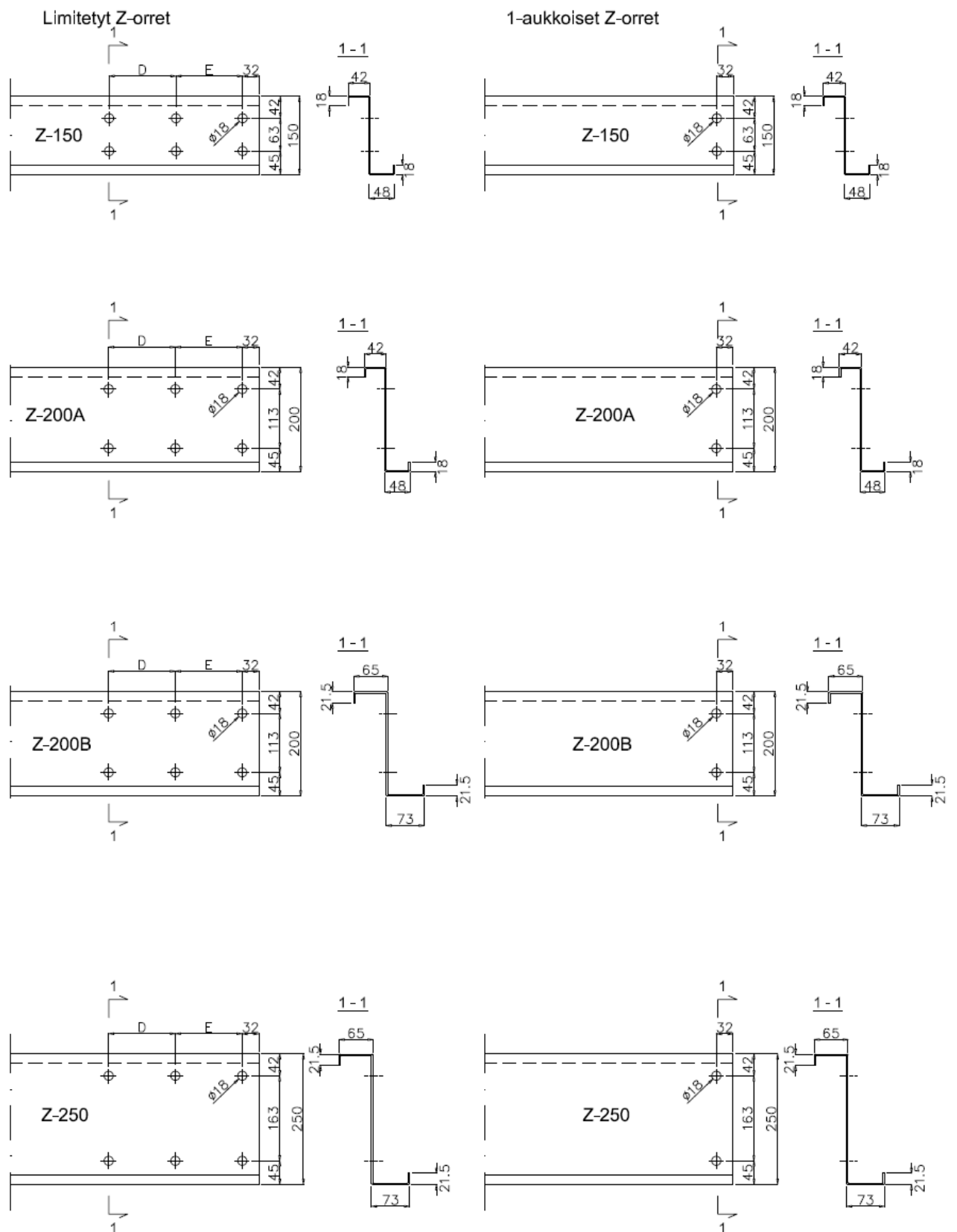
Kuva 3. Z-orsien vakioreijitykset.
