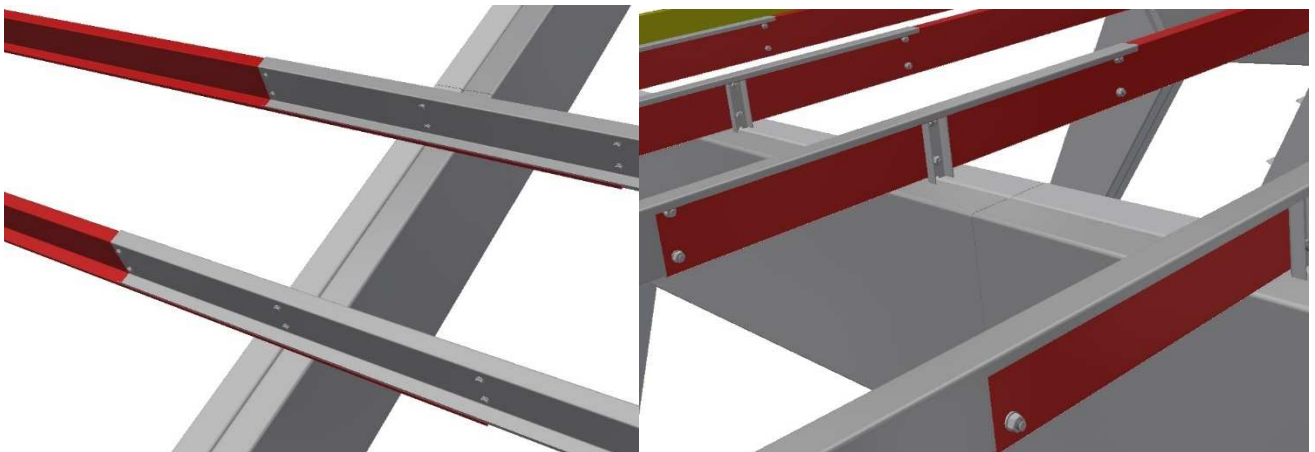
Kuva 12. Päittäin limitetty orsiliitos.
