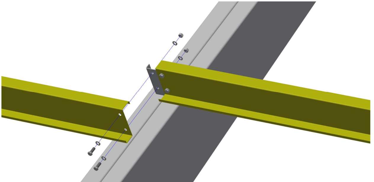
Kuva 15. Toisen orren kiinnitys epäjatkuvassa orsiliitoksessa.
