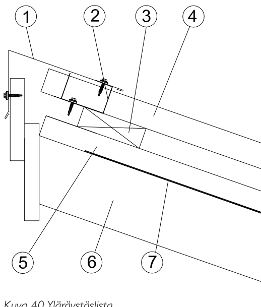
Kuva 40. Yläräystäslista
