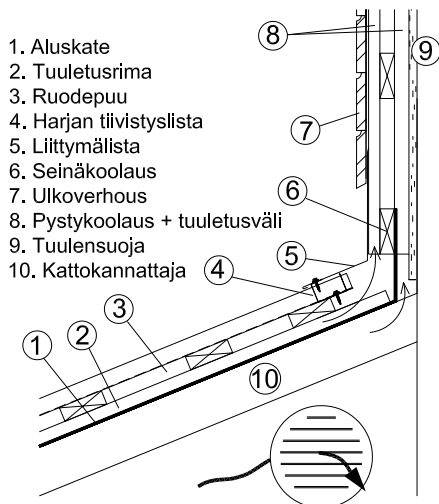
Kuva 35. Poikittainen rintataite
