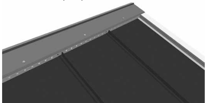
Kuva 34. Harjalistan kiinnitys.
