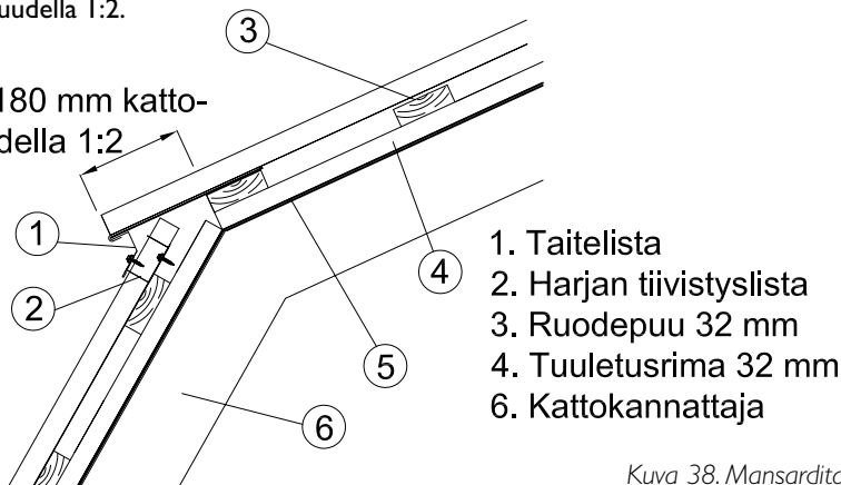
Kuva 38. Mansarditaite
