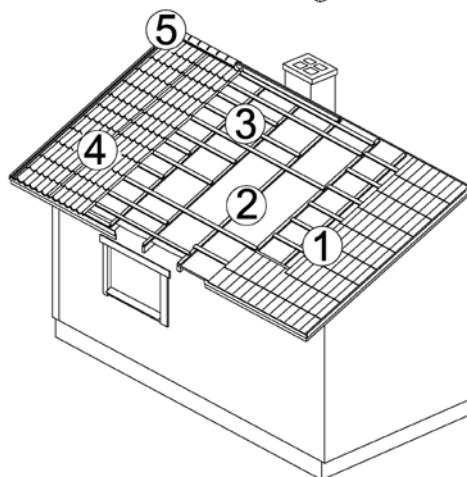
Kuva 47. Vanhan saumattun peltikaton saneeraus.
