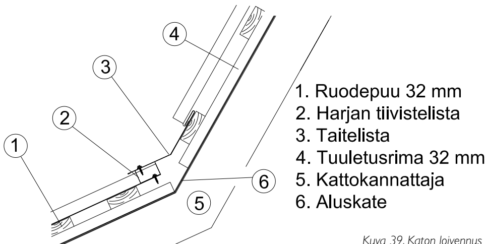
Kuva 39. Katon loivennus
