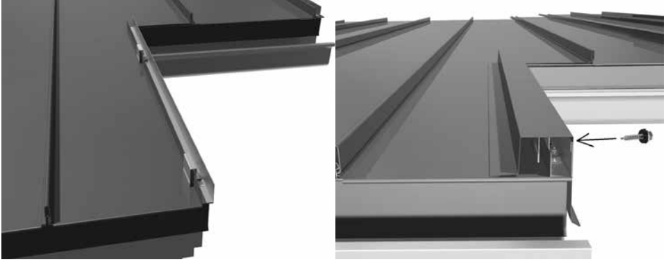
Kuva 28. Aluslista ja sivukiinnikkeet asennettuina Kuva 29. Päätylista kiinnitettynä
