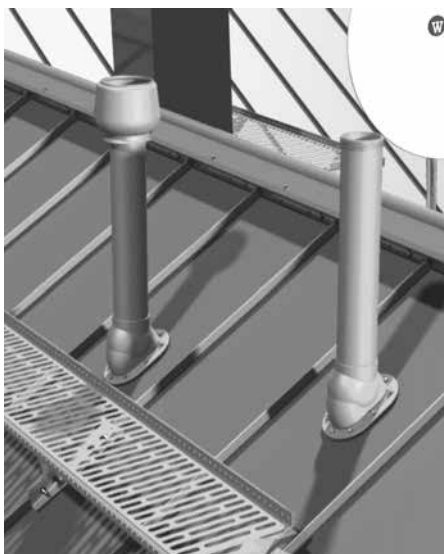
Kuva 41. Läpivientielementtien sijainti lappeella.
