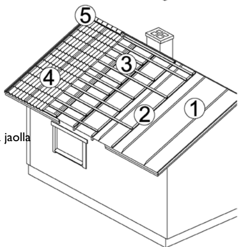
Kuva 48. Vanhan saumattun peltikaton saneeraus.
