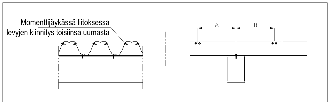
Kuva 7. Molempiin suuntiin limitetty momenttijäykä jatkos.
