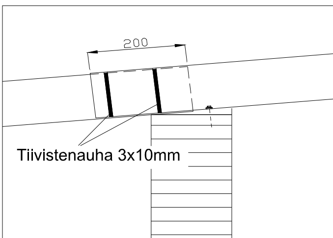
Kuva 11. Lämpöliikkeet salliva jatkolimitys.
