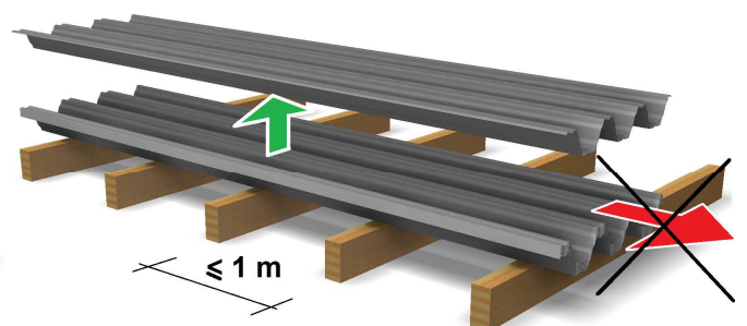
Kuva 1b. Levynippujen purku
