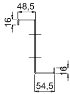
1 - 1 (t=1,2 mm)
