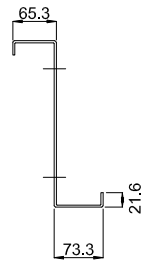
1 - 1 (t=1,5 mm)
