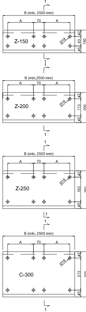
Sleeve-jatkoskappaleet
