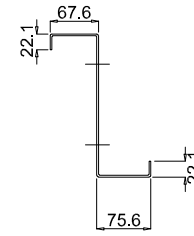
1 - 1 (t=2,5 mm)
