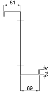
1 - 1 (t=1,5 mm)
