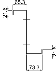
1 - 1 (t=1,5 mm)
