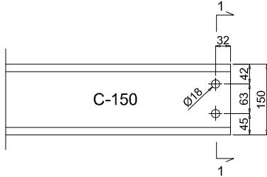
1-aukkoiset C-orret
