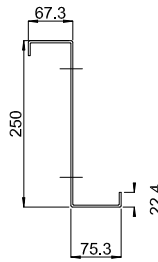
1 - 1 (t=2,5 mm)
