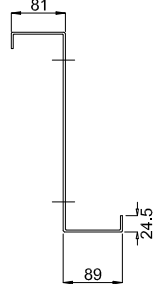
1 - 1 (t=1,5 mm)
