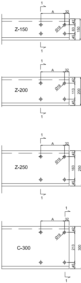
Sleeve-jatketut Z-orret
