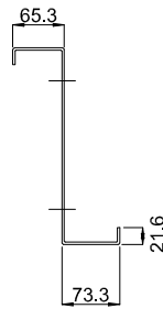
1 - 1 (t=1,5 mm)
