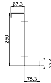
1 - 1 (t=2,5 mm)
