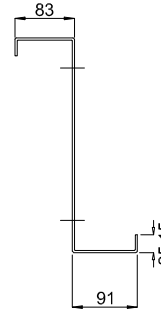
1 - 1 (t=2,5 mm)
