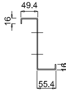
1 - 1 (t=1,5 mm)
