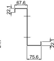
1 - 1 (t=2,5 mm)
