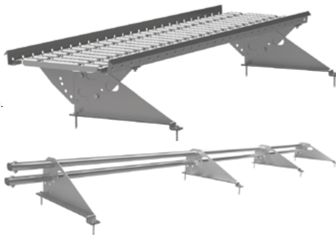
Lumieste on Suomen oloissa välttämätön tuote kulkureittien kohdalla. Kattosiltaja voidaan käyttää myös työtasojen ja porrasaskelmien rakentamiseen katolla.
