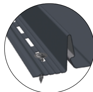
Urat varmistavat aina oikean ruuvien kiinnitys-kireyden
