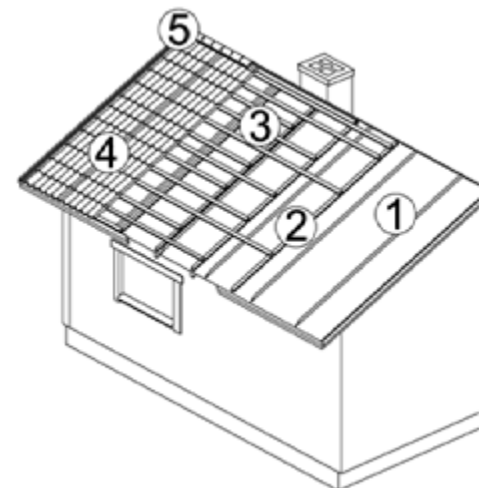
Kuva 56. Vanhan saumatun peltikaton saneeraus.
