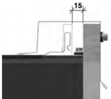
Kuva 13. Katelevyn etäisyys päädyistä
