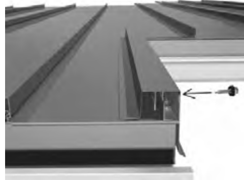
Kuva 29. Päätylista kiinnitettynä
