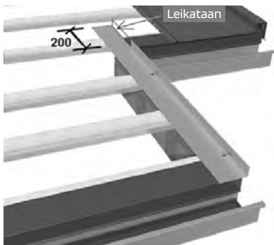
Kuva 26. Aluslista
