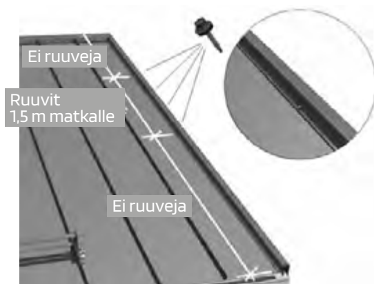
Kuva 24a. Päätylistan kiinnitys päätylautaan
