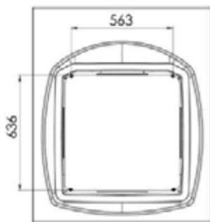
Kuva 40. Kiinnityspisteiden mitat
