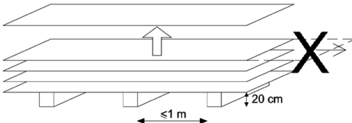
Kuva 1. Levyjen käsittely.
