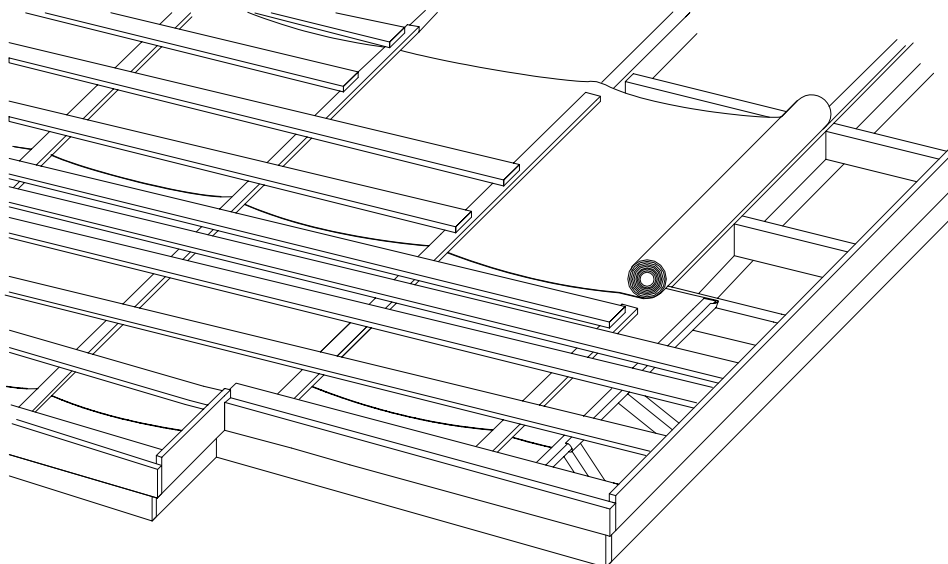
Kuva 7. Alusrakenne
