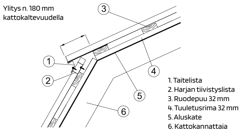
Kuva 36. Mansarditaite
