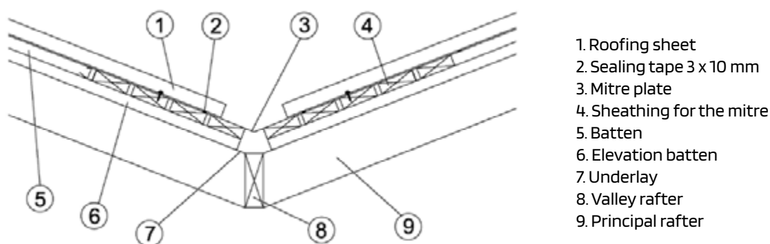
Figure 22. Inner mitre
