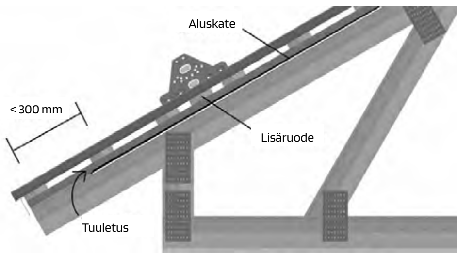
Kuva 9. Alaräystäs rakenne
