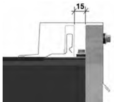
Kuva 13. Katelevyn etäisyys päädyistä
