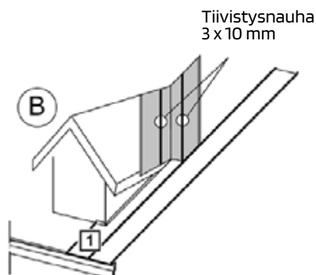
Kuva 23 B. Jiirilevyjen leikkaus ja jiiritiivisteiden kiinnitys
