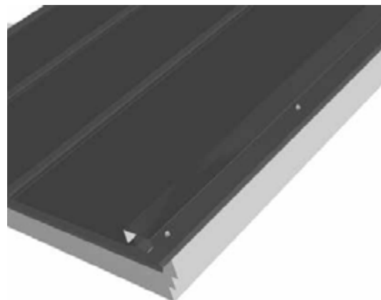
Kuva 24b. Päätylistan kiinnitys päätylautaan
