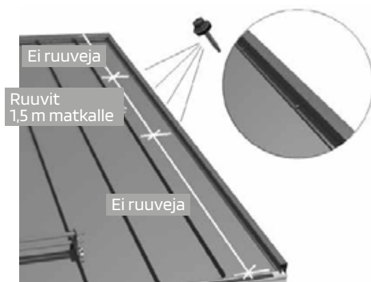
Kuva 24a. Päätylistan kiinnitys ruoteeseen
