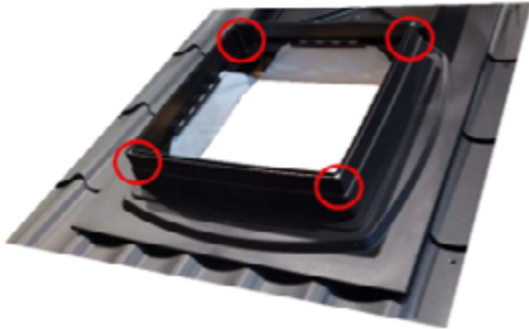
Kuva 47. Ruuvien paikat
