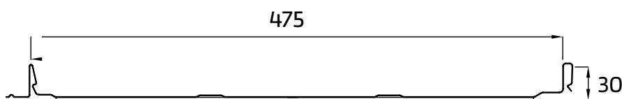
Kuva 4b. PROGANTTI J nimellis-poikkileikkausmitat SFS EN-508-1 toleranssien mukaan
