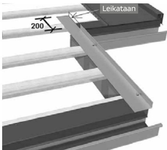
Kuva 26. Aluslista
