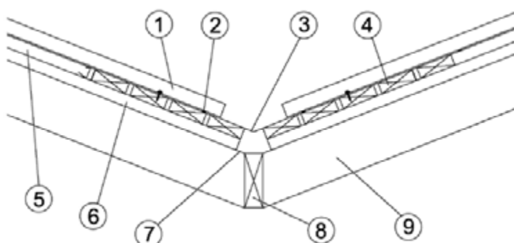
Figure 22. Inner mitre
