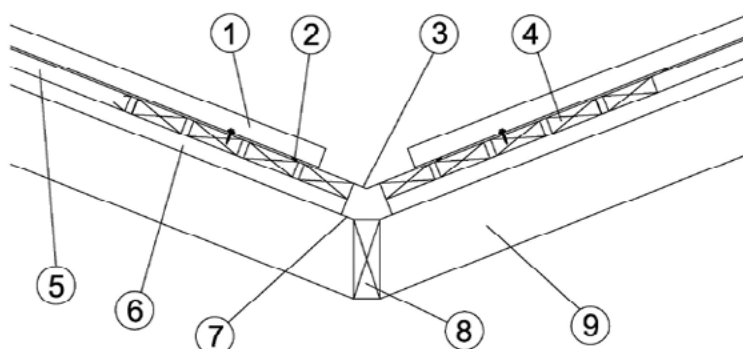
Figure 22. Inner mitre
